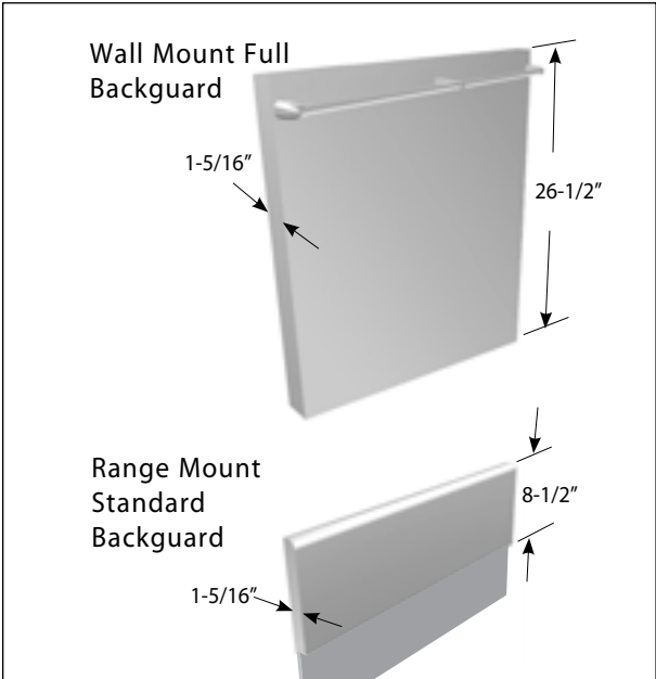
Fig.1 Backguards
