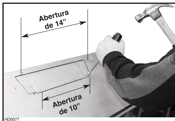
HD0077 Rompe la abertura vertical en la placa del ventilador
