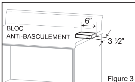
BLOC ANTI-BASCULEMENT
