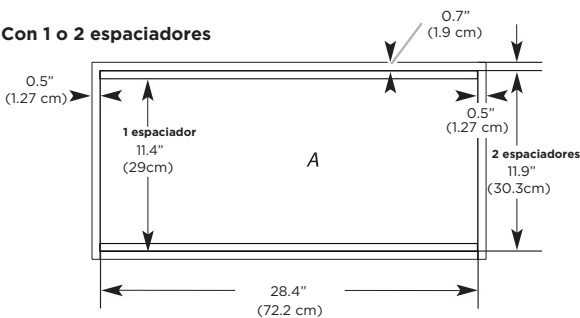
A. Corte inferior de gabinete
