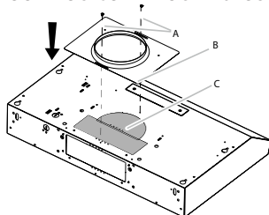
A. Tornillos .29 x .65 cm B. Placa de montaje 7" (17.8 cm) C. Precorte redondo
