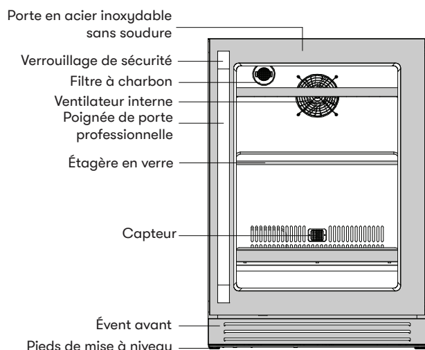
PRPB24C01CG avec porte et étagère en verre standard
