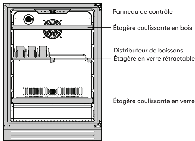
PRPB24C01CG sans porte et avec distributeur de boissons et étagère en verre rétractable
