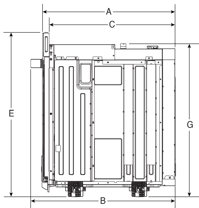
VUE LATÉRALE
