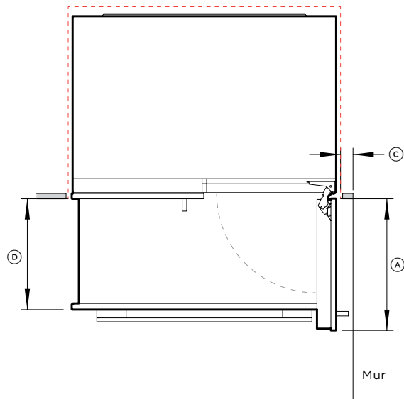
ACCÈS RÉDUIT À 90° À L'INTÉRIEUR
