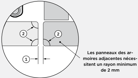
DÉTAIL 1
