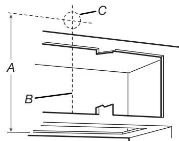
A. Mesure A B. Ligne centrale C. Ouverture rond de 6 1/4 po (15,9 cm)
