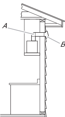
A. Conduit de diamètre 6 po (15,2 cm) pour décharge à travers le mur B. Bouche de décharge murale
