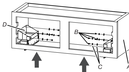
A. 36 po (91,4 cm) armoire B. Vis - 4,5 x 13 mm (8) C. Rondelles (facultatif) D. Support de montage (4) (Position pour 36 po [91,4 cm] armoire)
