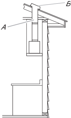
A. Conduit de diamètre 6 po (15,2 cm) pour décharge à travers le toit B. Bouche de décharge sur toit
