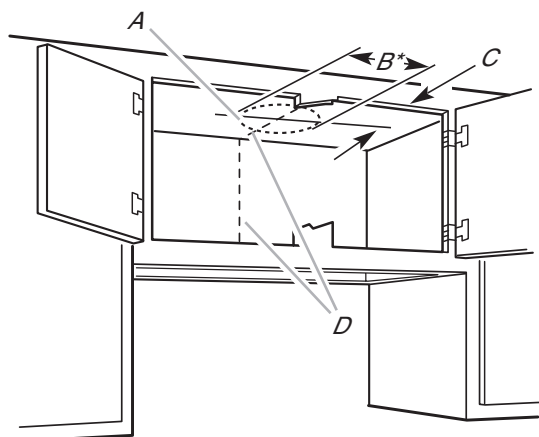
A. Ouverture B. Ø 6 1/4 po (15,9 cm) C. Ligne centrale de 7 1/2 po (19 cm) au devant de l'armoire D. Ligne centrale
