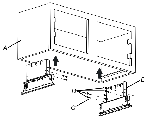
A. 30 po (76,2 cm) armoire B. Vis - 4,5 x 13 mm (8) C. Rondelles (facultatif) D. Support de montage (4) (Position pour 30 po [76,2 cm] armoire)
