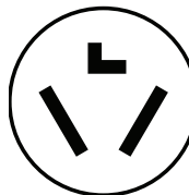
Tomacorriente de 3 hilos (10-30R)
