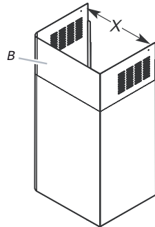
C. Tornillos de 4.2 x 8 mm D. Línea central
