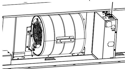
Instalación de la Ventilación Vertical
