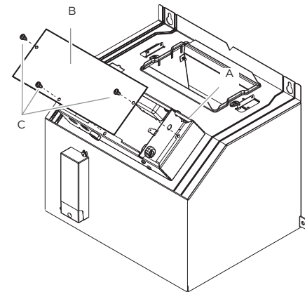
A. Precorte removible B. Cubierta de la caja eléctrica C. Caja eléctrica
