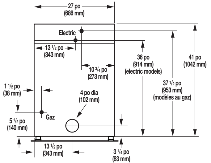
Vue arrière
