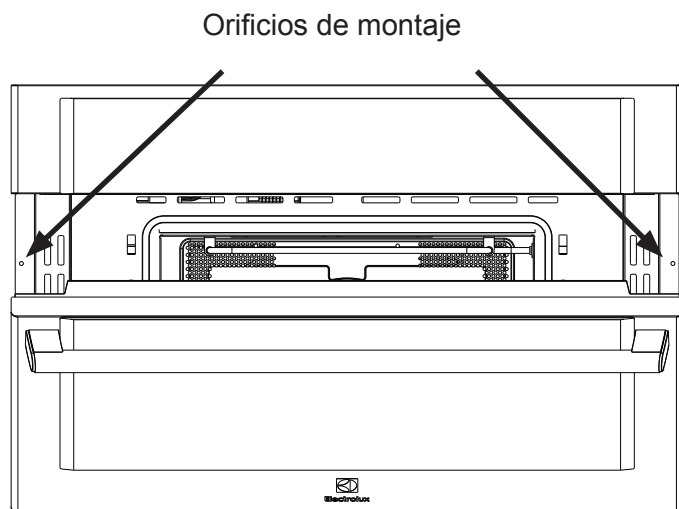
Figura 5: Orificios de tornillos
