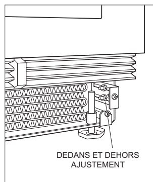
Réglage de la plaque de protection
