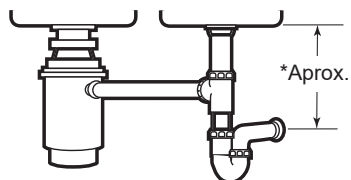
SALIDA EN EL EXTREMO CON RECIPIENTE DOBLE**
