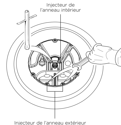
Brûleur double
