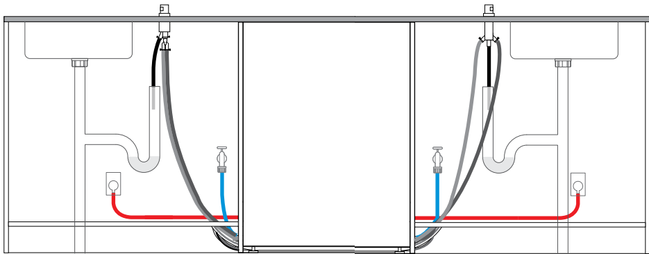
INSTALACIÓN DE ESPACIO DE AIRE INDIVIDUAL
