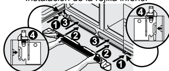
Instalación de la rejilla inferior
