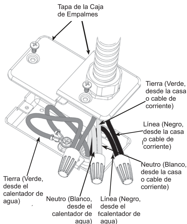
Ilustración de la Caja de Empalmes del Calentador de Agua
