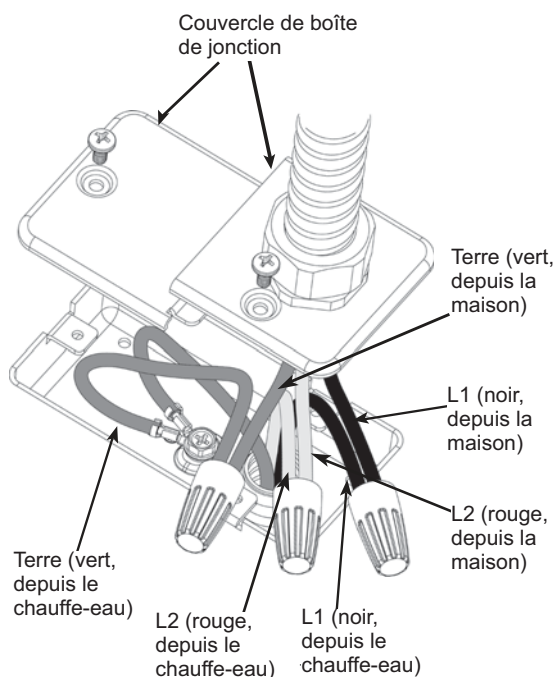
Illustration de la boîte de jonction du chauffe-eau
