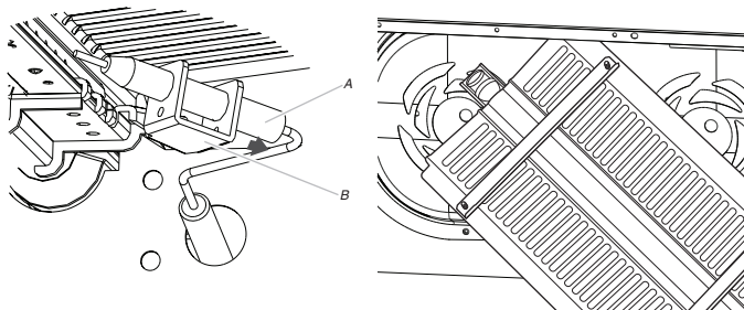
A. Tome el electrodo de aquí B. Soporte Quemador para asar colgando en la parte trasera del horno
