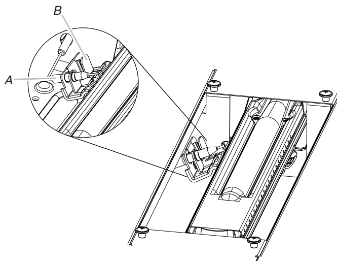
A. Électrode du brûleur de cuisson au four
