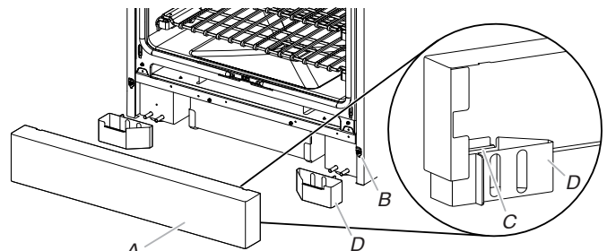
A. Plinthe B. Onglet de plinthe C. Fente de plinthe D. Pieds
