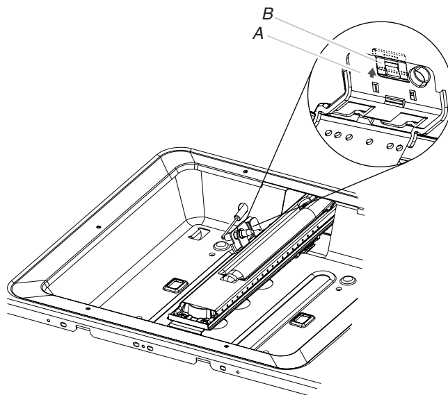
A. Soporte del electrodo del quemador para hornear del horno B. Broche del soporte del electrodo
