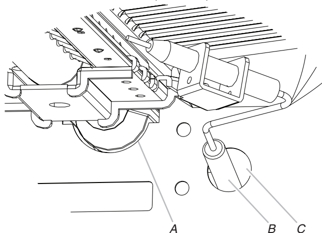
A. Agujero del orificio del quemador para asar B. Electrodo del quemador para asar C. Agujero del electrodo del quemador para asar
