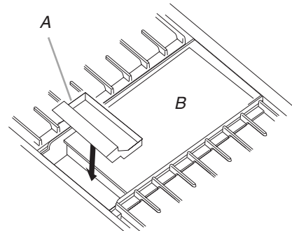
A. Bandeja de goteo de la plancha B. Plancha
