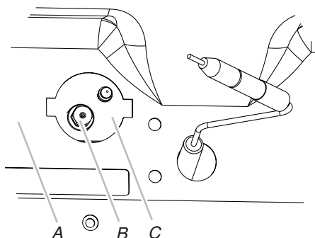
A. Arrière du four B. Gicleur du brûleur de cuisson au gril C. Orifice du gicleur de brûleur de cuisson au gril
