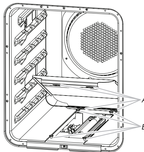
A. Trous de montage (encoches allongées) de vis à épaulement
