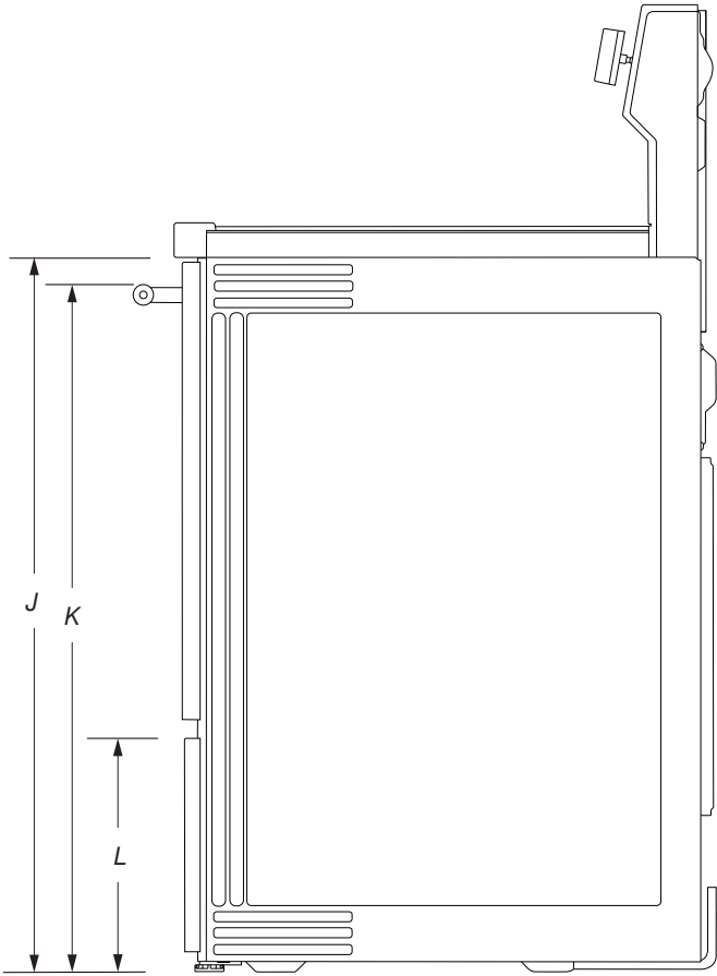
VUE LATÉRALE
