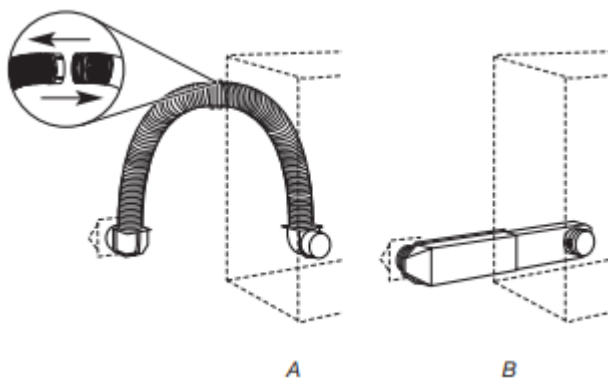
A. Installation au-dessus de la sècheuse (également offerte avec un coude décalé) B. Installation en périscope
