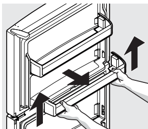
Porte bin
