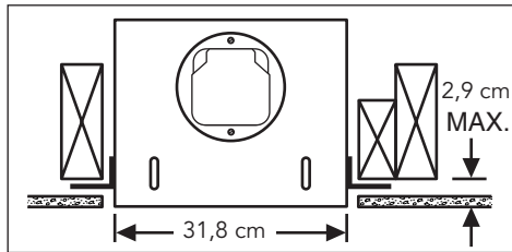
Abrazaderas de montaje en la posición ajustada en fábrica. (La salida queda paralela a la viguetas) (Estructura nueva )
