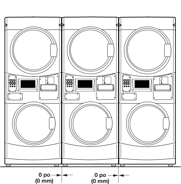
Distances de dégagement latéral
