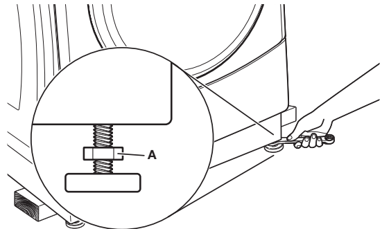
A. Contre-écrou
