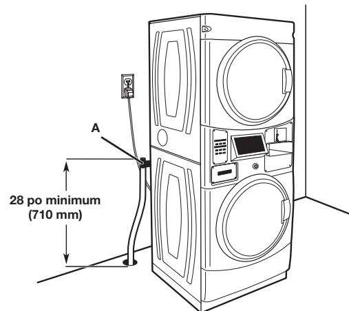
A. Brise-siphon
