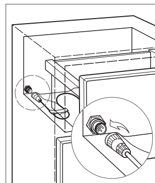
Cable de control (modelo de cajón)
