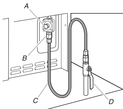
A. Détendeur B. Raccord d'adaptation C. Raccord flexible D. Robinet d'arrêt manuel
