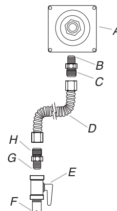
A. Détendeur B. Utiliser un composé d'étanchéité des tuyauteries C. Adaptateur (doit comporter un filetage mâle de 1/2" [12,7 mm]) D. Raccord flexible E. Robinet d'arrêt manuel F. Tuyau de gaz de 1/2" ou 3/4" (12,7 mm ou 19 mm) G. Utiliser un composé d'étanchéité des tuyauteries H. Adaptateur
