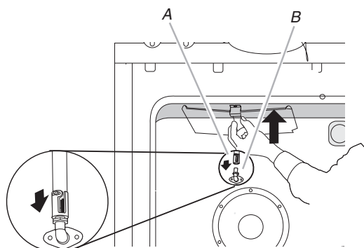
A. Gicleur de brûleur de grill B. Grille de la lèche-frite
