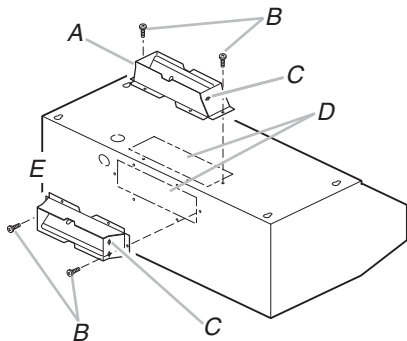
A. Ventilación superior B. Tornillos para lámina metálica C. Pasador de la bisagra D. Discos removibles de la ventilación E. Ventilación trasera
