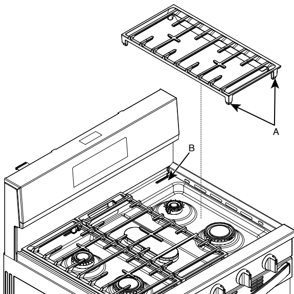
A. Butoir B. Indentations d'alignement
