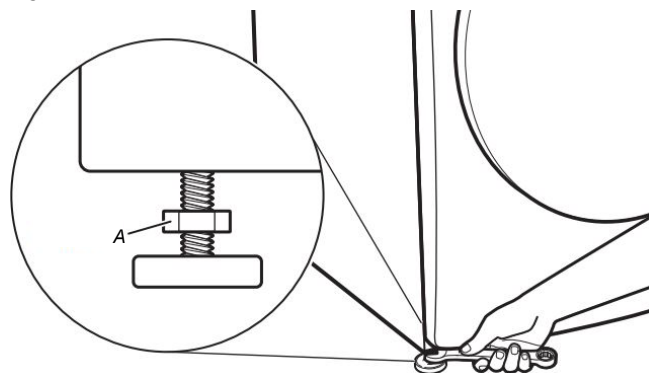
A. Contre-écrou
