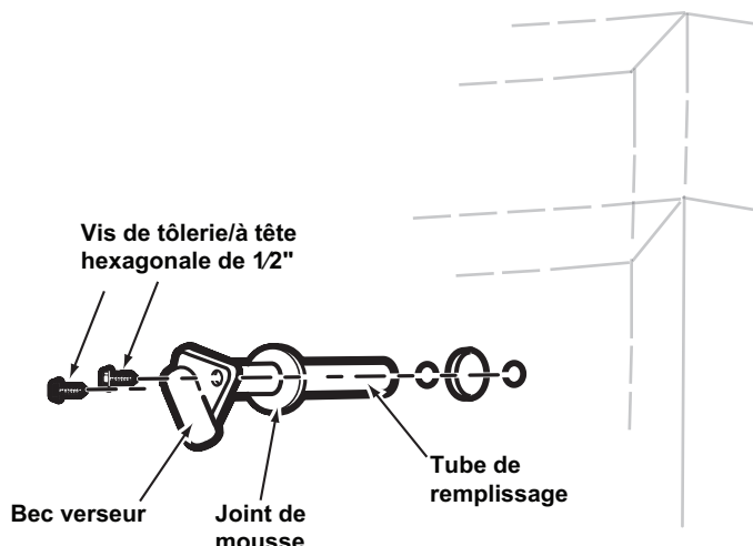
Installation de l'ensemble tube de remplissage/joint (Modèles à congélateur en bas - 14 à 18 pi 3 )
