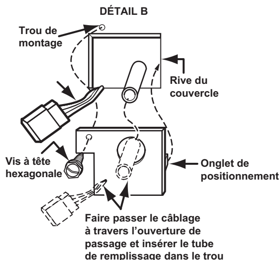
Réinstallation du couvercle du logement du câblage
