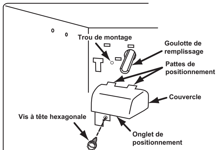
Dépose du couvercle du logement du câblage - modèle avec goutte de remplissage
