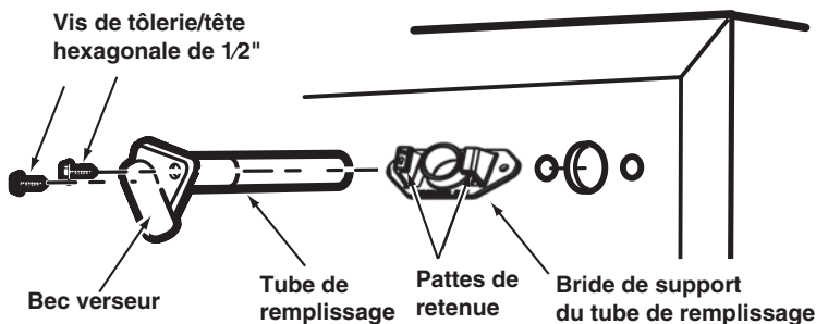
Installation de l'ensemble tube de remplissage/bride de support du tube de remplissage (modèles de 11 pi 3 )
