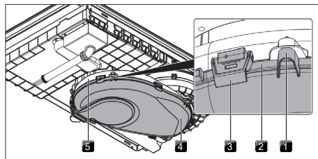
Fig. 9.2 Carcasa de conducción del aire
