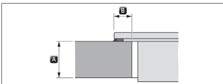
Fig. 11.11 Dimensiones de cobertura para montaje superpuesto
