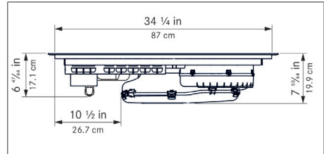
Fig. 5.5 Vue avant
