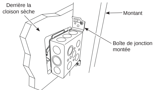
VUE ARRIÈRE
