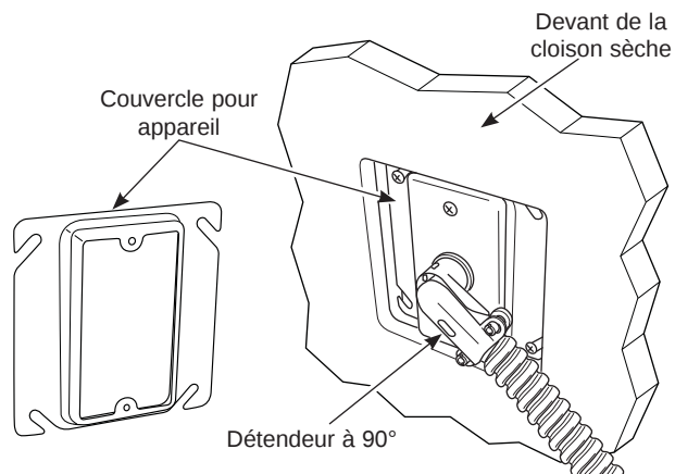
VUE AVANT
