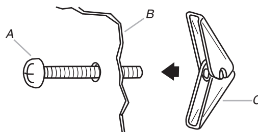
A. Vis à tête ronde de 3/16-24 x 3 po
