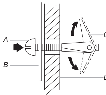
A. Vis à tête ronde de \frac{3}{16} -24 x 3 po B. Plaque de montage C. Écrou articulé à ressort D. Panneau de gypse
