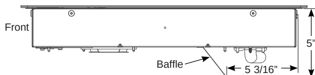
Baffle dimensions
