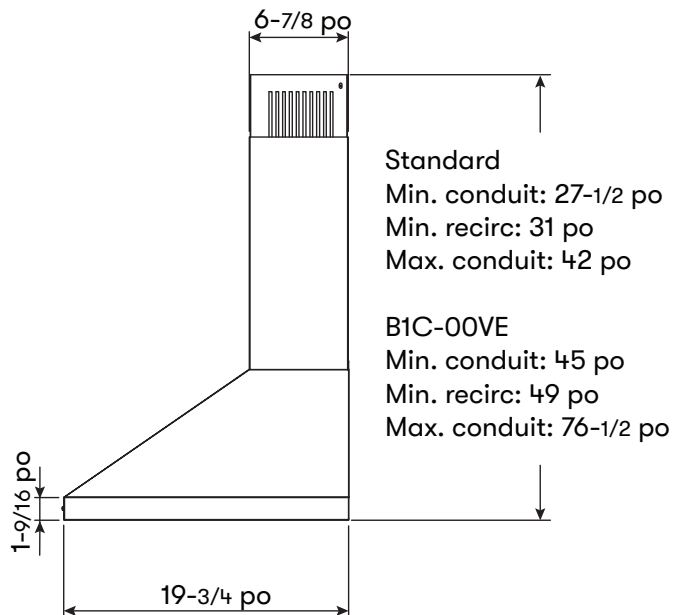
CÔTÉ
