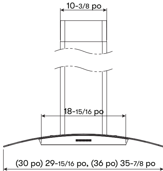
DEVANT
