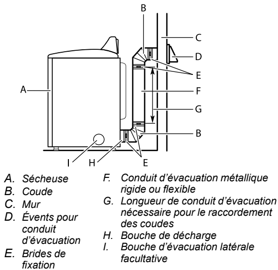
Installation au-dessus de la sècheuse (également offerte avec un coude décalé) Installation en périscope
