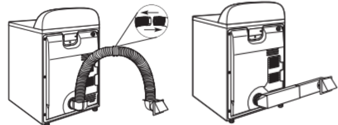
Instalación en la parte superior (también está disponible con un codo de desviación) Instalación de periscopio
