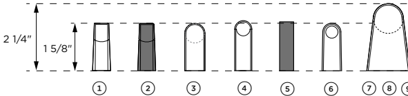
PERFILES
