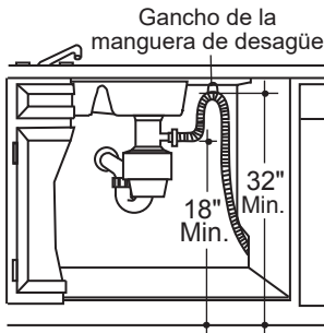
Instalación del eliminador de desechos
