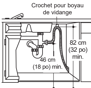
Installation avec raccord en T
