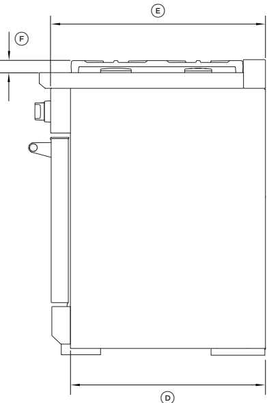
PROFIL
