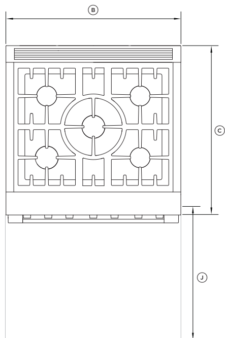
EN PLAN
