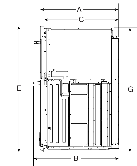
VUE LATÉRALE
