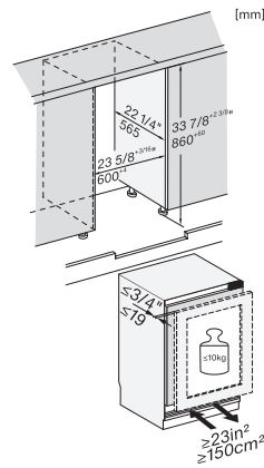
KWTUS7172F, Built-under, Einbauskizze, Nischenmaß (installation drawings) (US, CA)
