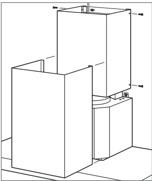
Installez la cheminée téléscopique
