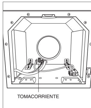
Tomacorriente de la campana
