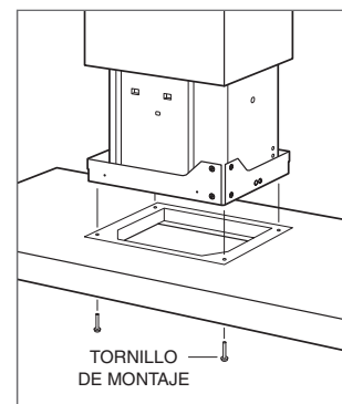
Instale la campana
