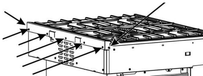
Figure 1: Tornillos de la moldura, estufa de dos combustibles
