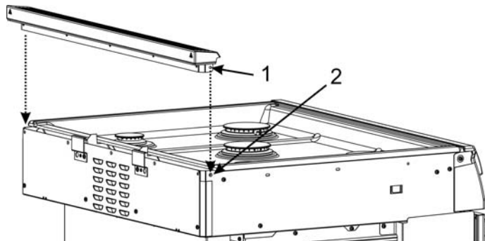
Figure 2 : Positionnement de la garniture d'îlot
