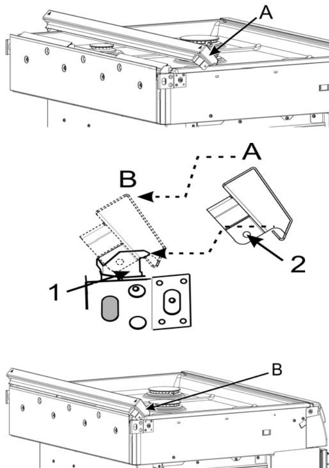
Figura 5: Colocación 1 de la moldura para islas
