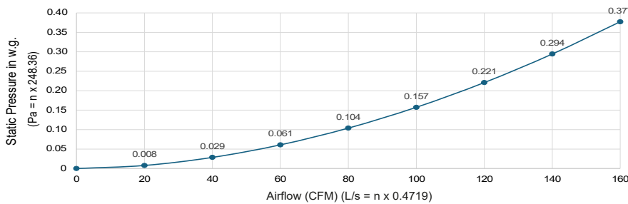
RENDIMIENTO DEL FLUJO DE AIRE A LA SALIDA
