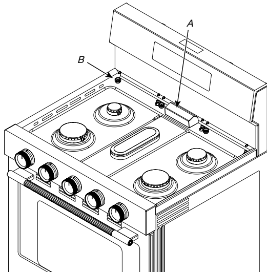
A. Couvercle de l'évent central du four B. Éléments de positionnement
