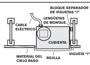
Montaje de la cubierta en viguetas "I" .
