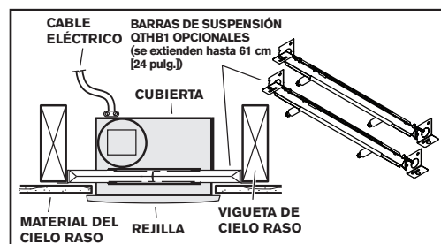
Montaje de la cubierta en viguetas .
