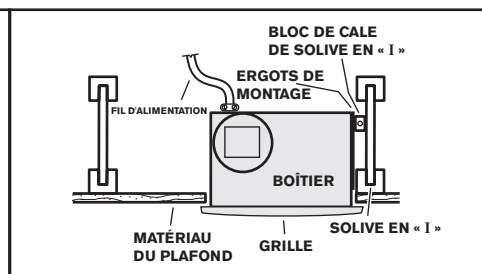
Boîtier fixé aux solives en « I »
