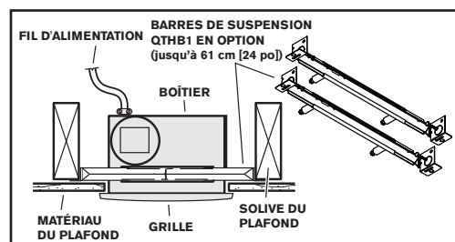
Boîtier fixé aux solives .
