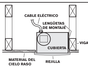
Montaje de la cubierta a la viga .
