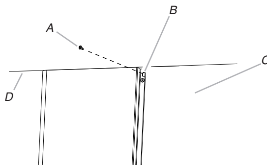
A. Vis de 3,5 x 6,5 mm B. Trous allongés (2) C. Partie supérieure des cache-conduits D. Plafond
