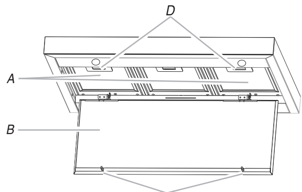
A. Filtres métalliques
